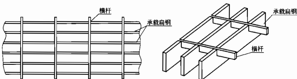
图2 压锁钢格板
