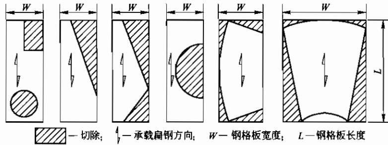
图9 异形钢格板
