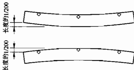
图 6 纵向弯曲
