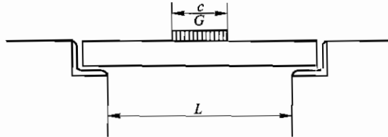
图 B. 5 轮荷载模型
