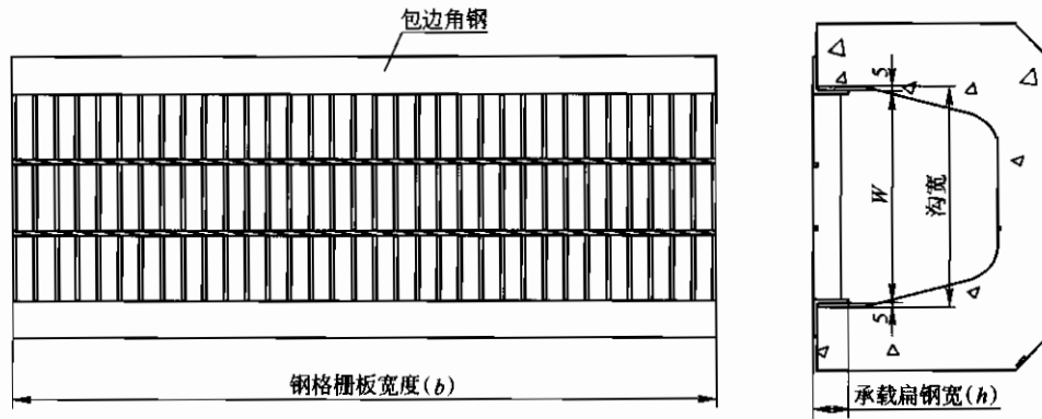
图 B.3 GU 型沟钢格栅沟盖
