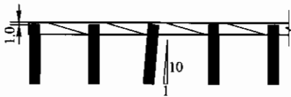
图 4 承载扁钢、横杆的偏差
